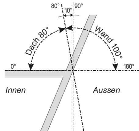
Beispiel: geneigte Fassade
