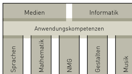
Abbildung 1: Struktur Modullehrplan
