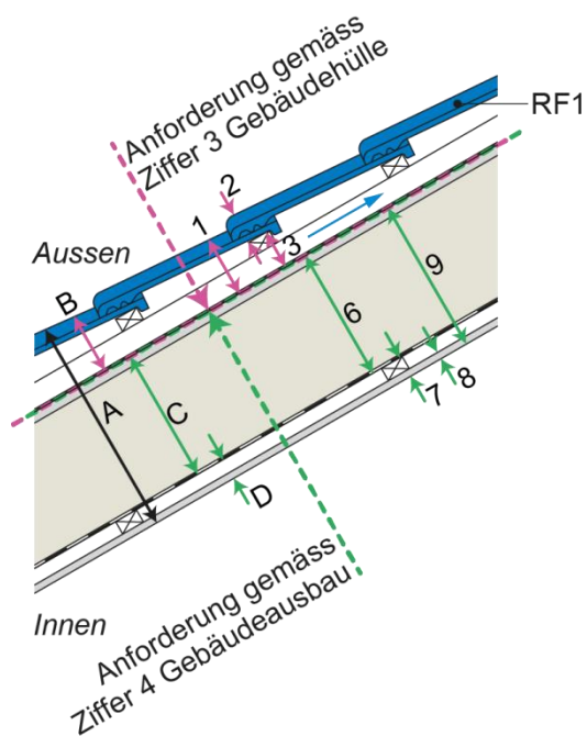
Variante 1, Warmdach einfach belüftet
